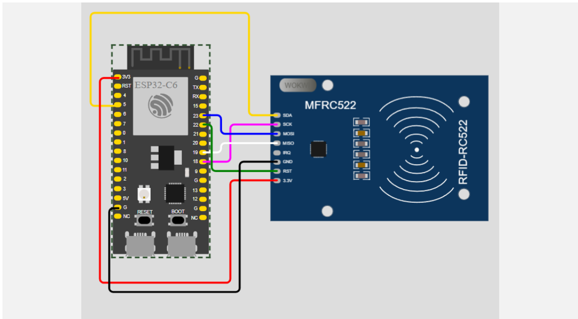
conexión física de módulo RFID RC522 a ESP 32 C6, usando simulador WOKWI
